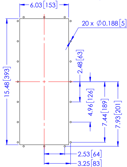
Mounting Cutout, Découpe d'Installation, Einbauausschnitt, Installazione Ritaglio
